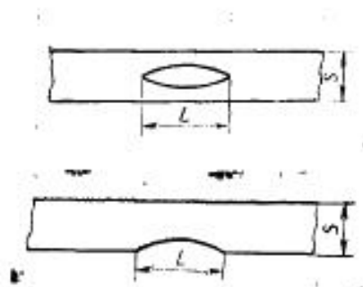
Рисунок 2 — Длина дефекта
